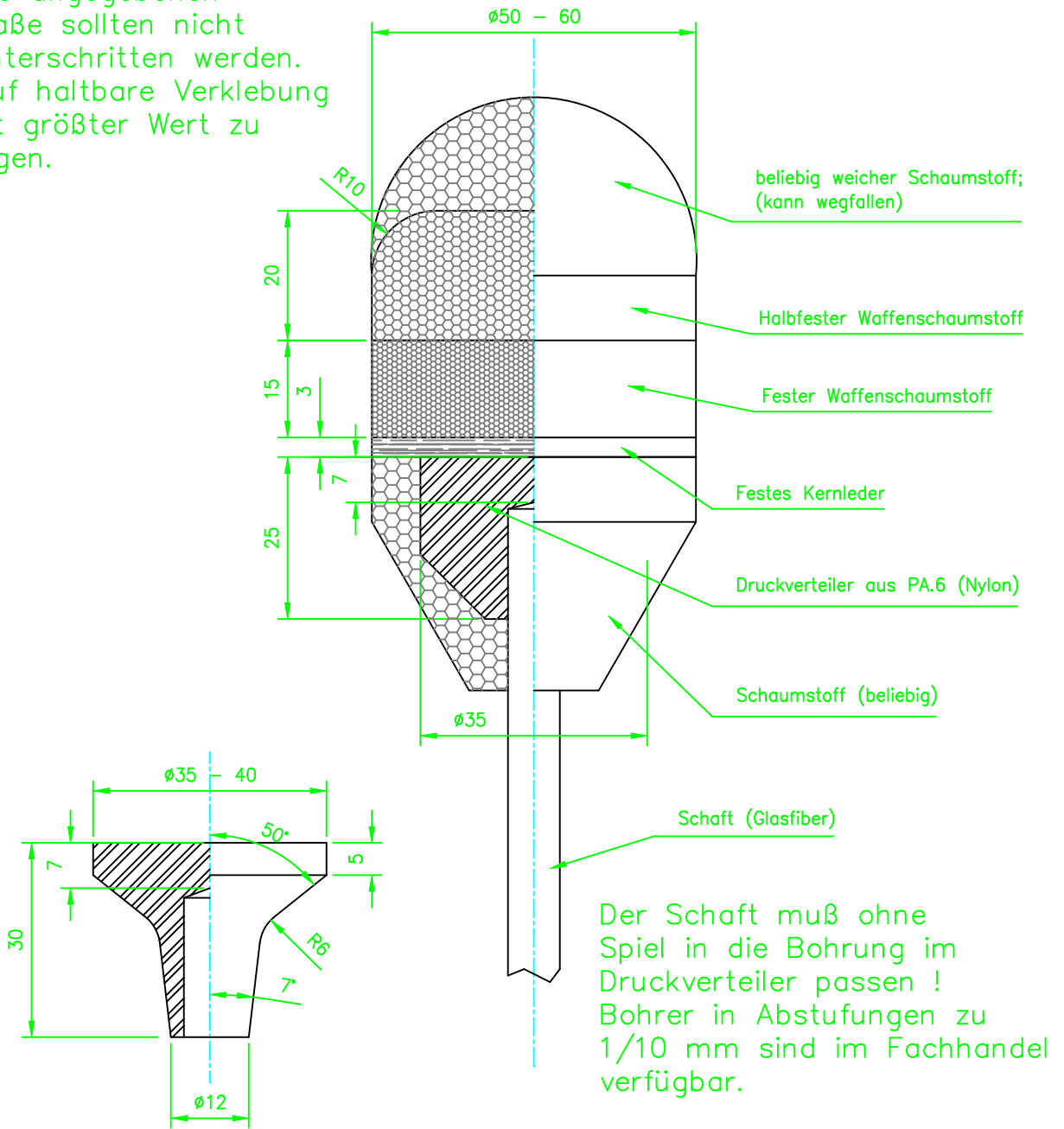
Alternative Form eines Druckverteilers (weniger Gewicht)
